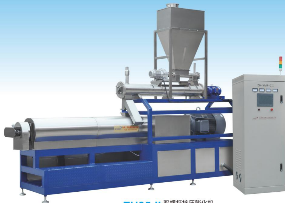
ZH85-II 双螺杆挤压膨化机 Double-screw Extruder
